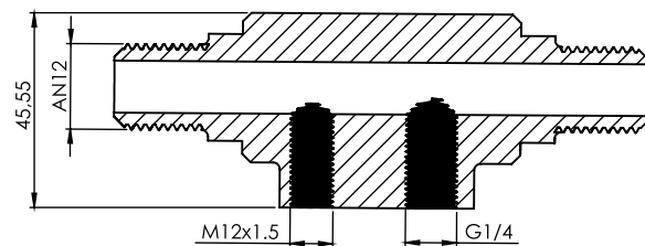
SECCIÓN B-B
